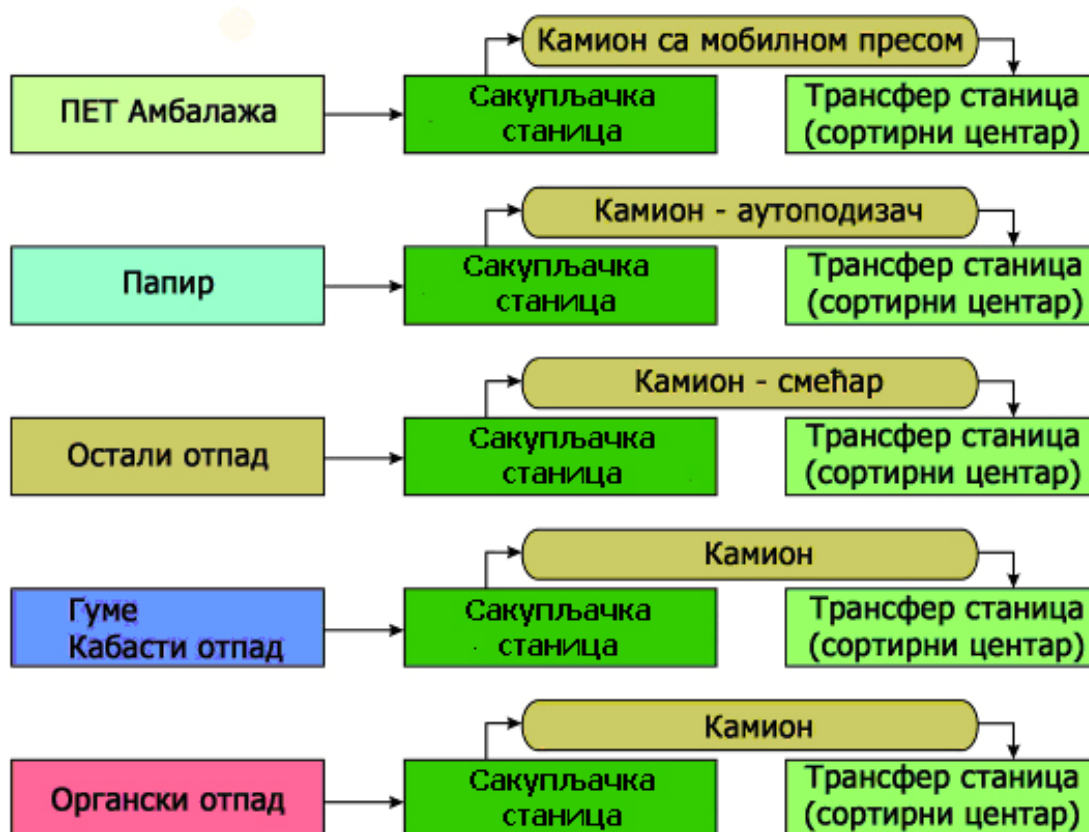
Шема 7 - Шематски приказ сакупљања и транспорта сепарисаног отпада за градско насеље
