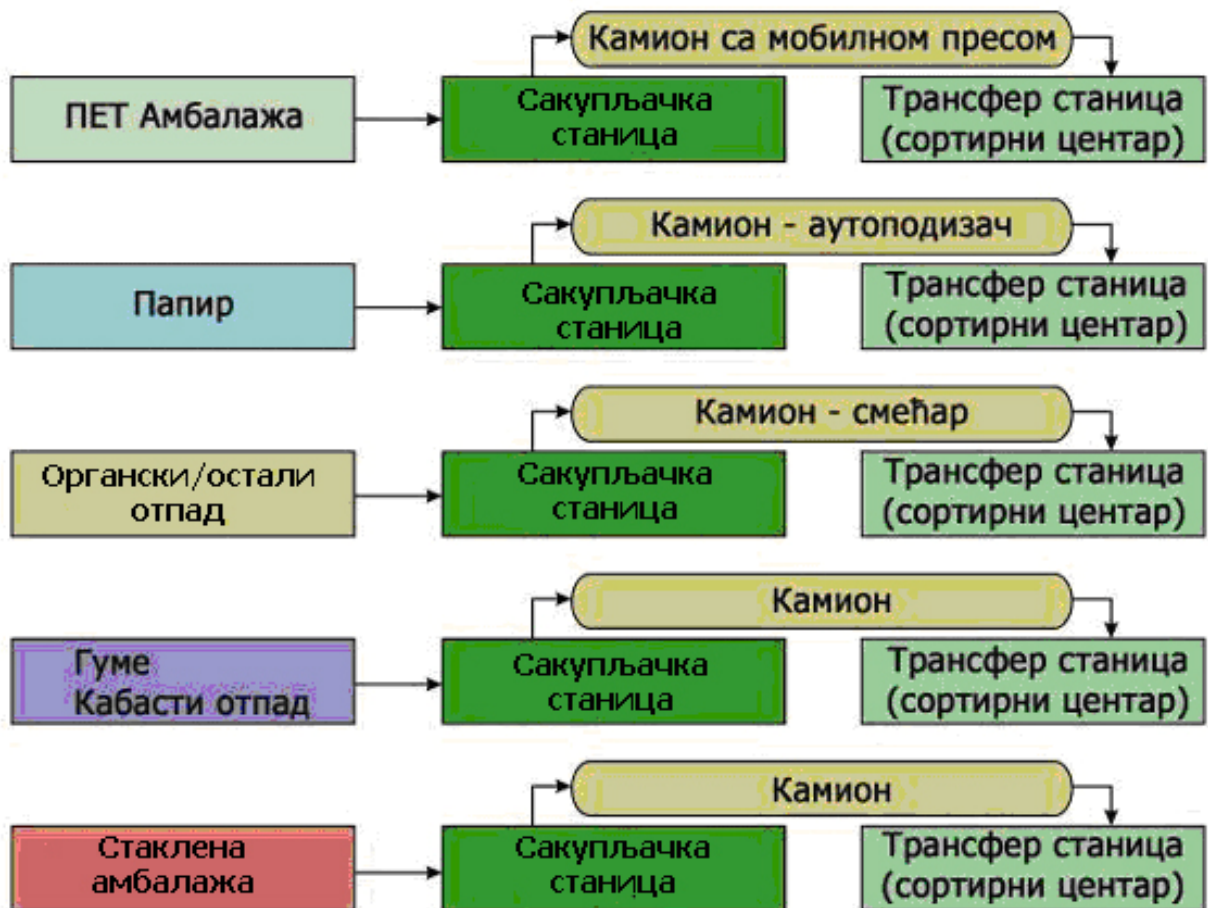
Шема 10 - Шематски приказ сакупљања и транспорта сепарисаног отпада за села III категорије
