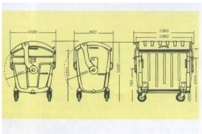
Слика 31 - Типичан контејнер запремине 1,1 m 3
